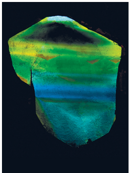
Karte Nr. 069 Dünnschliff, Afghanistan
